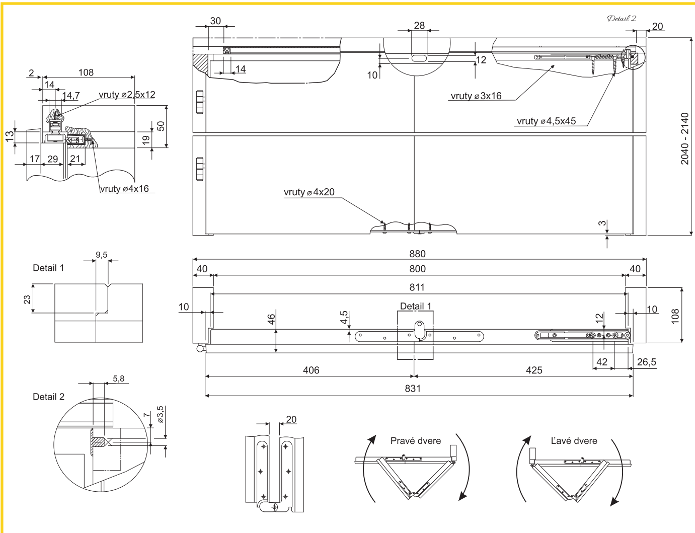
Otvárací mechanizmus
