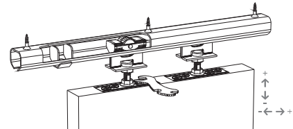
Nastavenie a fixácia dverí
