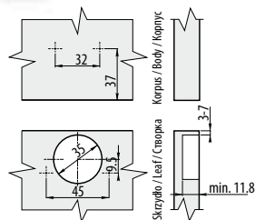
Wymiary montażowe / Mounting dimensions / Монтажные размеры
