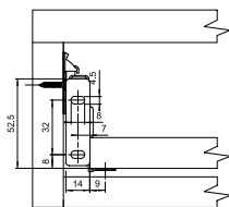
Wymiary montażowe frontów Mounting dimensions of fronts Монтажные размеры фронтальных панелей
