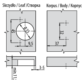
Wymiary montażowe / Mounting dimensions / Монтажные размеры
