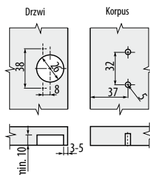
Wymiary montażowe / Mounting dimensions / Монтажные размеры
