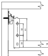
Wymiary montażowe ścianki tylnej Back wall mounting dimensions Монтажные размеры задней панели
