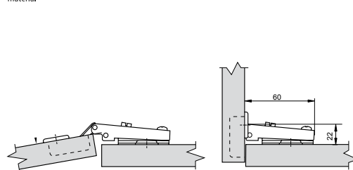
Drzwi otwarte / Door opened Открытые дверцы
