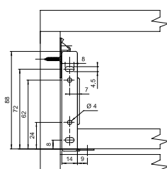
Wymiary montażowe frontów Mounting dimensions of fronts Монтажные размеры фронтальных панелей
