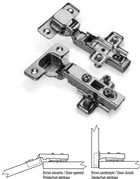
Wymiary montażowe / Mounting dimensions / Монтажные размеры
