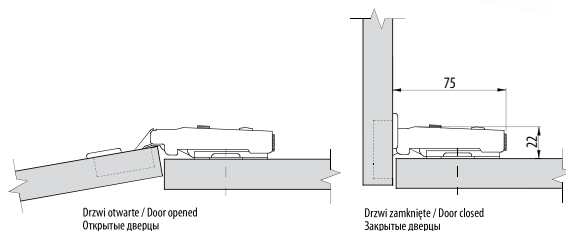
Wymiary montażowe / Mounting dimensions / Монтажные размеры
