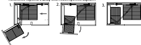
Położenie kosza w szafce. Wersja lewa / Bin position in the cupboard. Left-side version Положение корзины в шкафчике. Левосторонний вариант.
