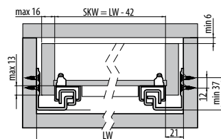
SKW - wewnętrzna szerokość szuflady / internal drawer width / внутренняя ширина ящика LW - wewnętrzna szerokość szafki / internal cabinet width / внутренняя ширина шкафчика
