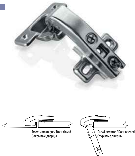
Wymiary montażowe / Mounting dimensions / Монтажные размеры
