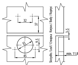
Wymiary montażowe / Mounting dimensions / Монтажные размеры
