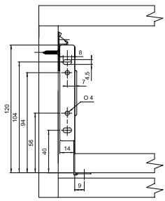
Wymiary montażowe frontów Mounting dimensions of fronts Монтажные размеры фронтальных панелей
