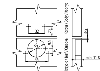
Wymiary montażowe / Mounting dimensions / Монтажные размеры
