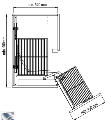
Położenie kosza w szafce. Wersja prawa / Bin position in the cupboard. Right-side version Положение корзины в шкафчике. Правосторонний вариант
