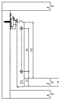
Wymiary montażowe ścianki tylnej Back wall mounting dimensions Монтажные размеры задней панели
