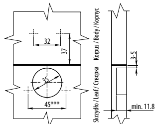
Wymiary montażowe / Mounting dimensions / Монтажные размеры
