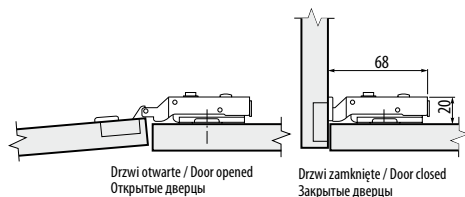
Wymiary montażowe / Mounting dimensions / Монтажные размеры
