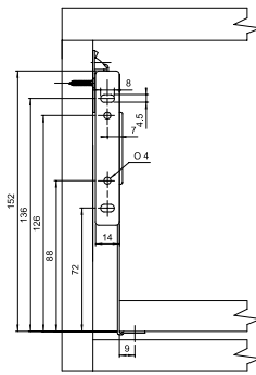
Wymiary montażowe frontów Mounting dimensions of fronts Монтажные размеры фронтальных панелей
