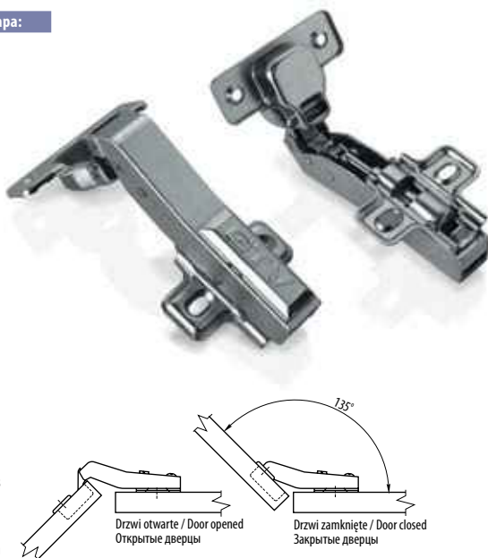
Wymiary montażowe / Mounting dimensions / Монтажные размеры
