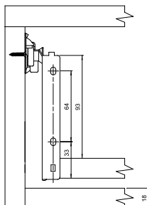
Wymiary montażowe ścianki tylnej Back wall mounting dimensions Монтажные размеры задней панели
