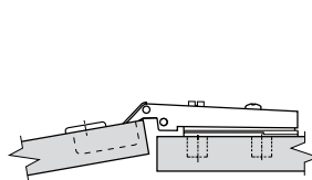
Drzwi otwarte / Door opened Открытые дверцы
