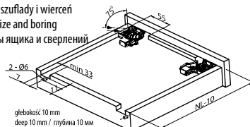
Standardowa szuflada / Standard drawer / Стандартный ящик, LT min = NL+3 LT - wewnętrzna głębokość szafki / internal cabinet depth / внутренняя глубина шкафчика
