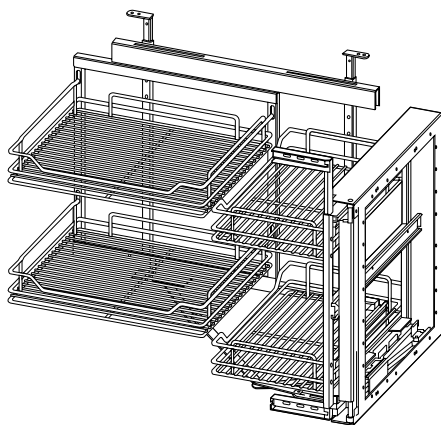
Położenie kosza w szafce. Wersja prawa / Bin position in the cupboard. Right-side version Положение корзины в шкафчике. Правосторонний вариант
