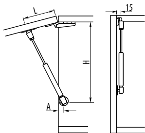
Drzwi wpuszczane / Flush door / Внутренние дверцы
