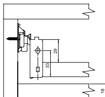
Wymiary montażowe ścianki tylnej Back wall mounting dimensions Монтажные размеры задней панели
