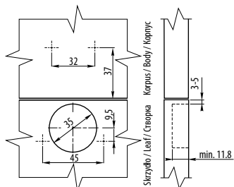
Wymiary montażowe / Mounting dimensions / Монтажные размеры
