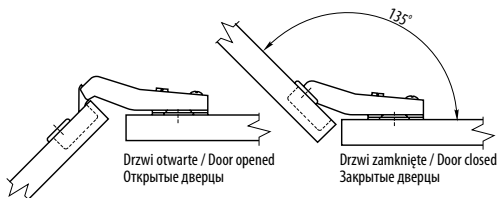
Wymiary montażowe / Mounting dimensions / Монтажные размеры
