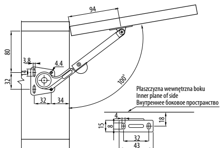
Drzwi nakładane 100° / Lift-off door 100° / Наружные дверцы 100°
