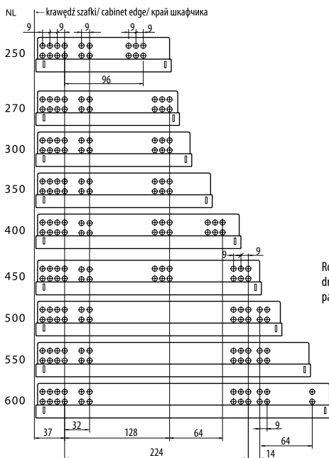
Wewnętrzna szuflada / Inner drawer / Внутренний ящик, LT min = NL+21
