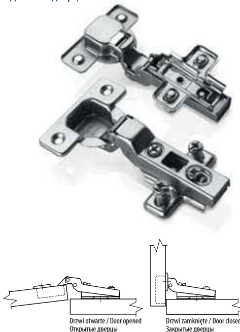
Wymiary montażowe / Mounting dimensions / Монтажные размеры
