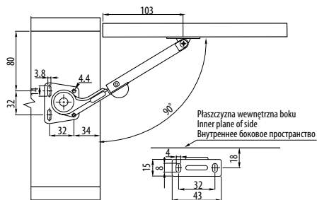
Drzwi nakładane 90° / Lift-off door 90° / Наружные дверцы 90°
