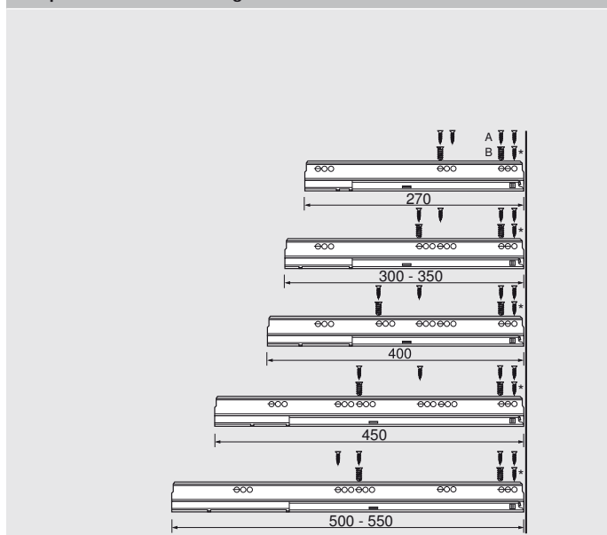
Korpusová lišta 558 – 30 kg
