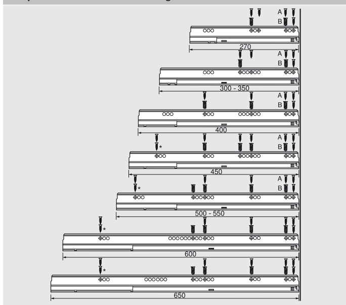
Korpusová lišta 559T – 20/30/50 kg
