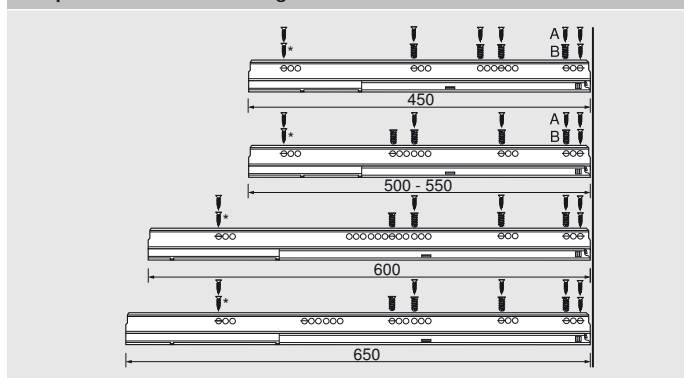
Korpusová lišta 559B – 50 kg
