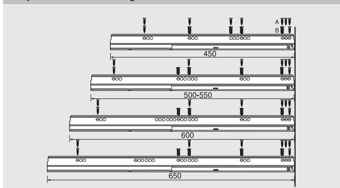
Korpusová lišta 556 – 65 kg
