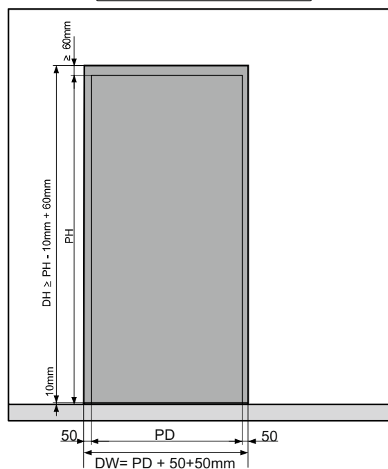
POLOHA DVERÍ PRI ZATVORENÍ
