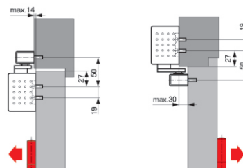
Možnosti montáže
