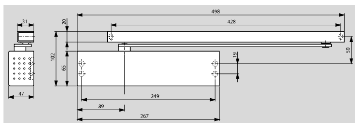
Možnosti montáže
