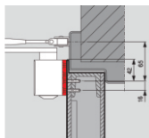
Možnosti montáže
