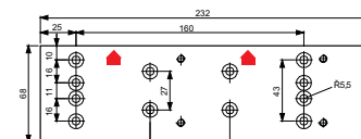
Montážna platnička
