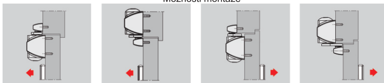
Rozdielná montáž pri sile EN 3 a EN 4
